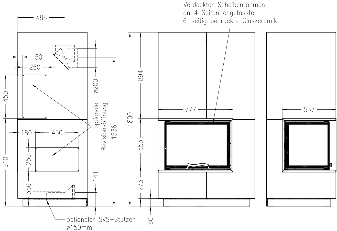
Draufsicht M~1:20
