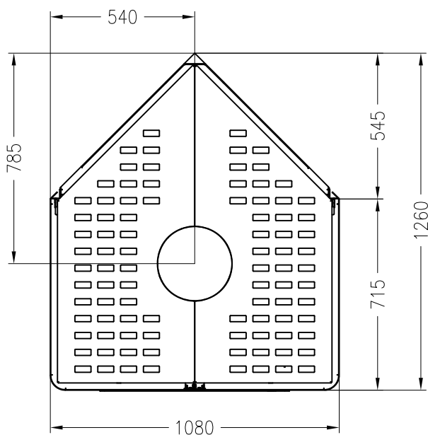
Draufsicht M~1:20
