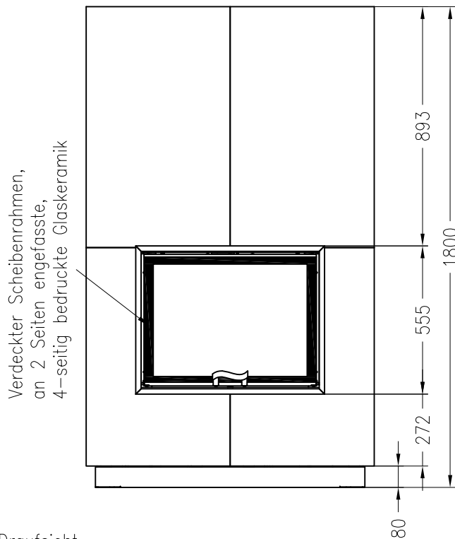
Draufsicht M~1:20
