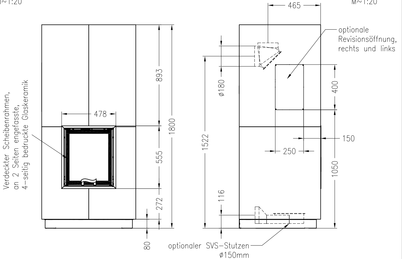
Draufsicht M~1:20
