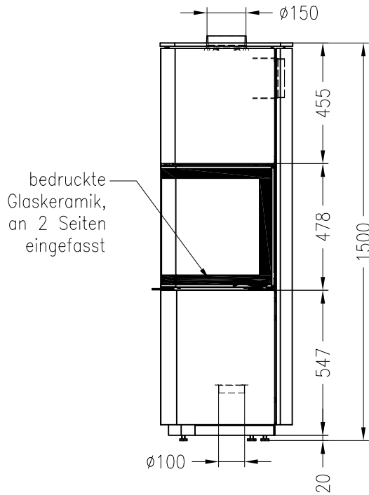
Vorderansicht M~1:20
